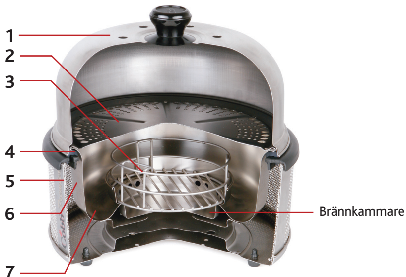
4 Låsringar 5 Yttre gjutning
